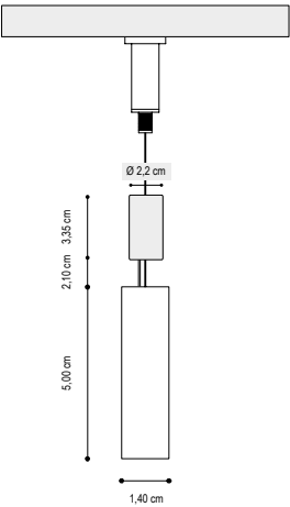
SEZIONE PROFILO/PROFILE SECTION
