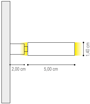
SEZIONE PROFILO/PROFILE SECTION
