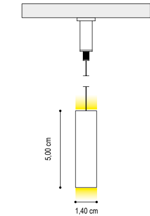
SEZIONE PROFILO/PROFILE SECTION
