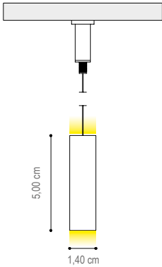
SEZIONE PROFILO/PROFILE SECTION
