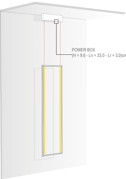
APOTEMA CON BOX APOTEMA WITH POWER SUPPLY BOX
