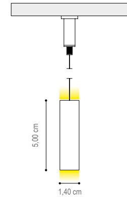
SEZIONE PROFILO/PROFILE SECTION
