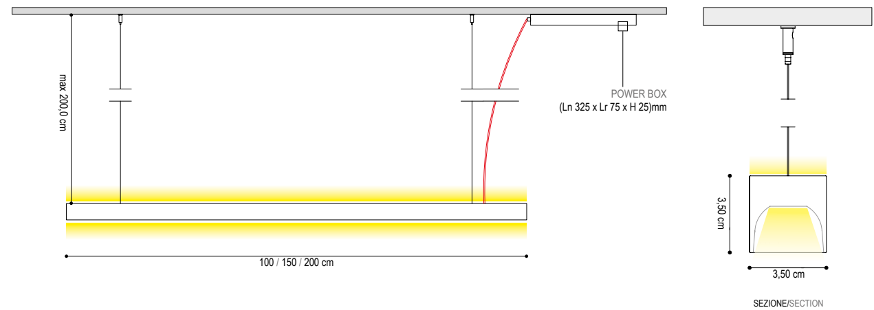
CARATTERISTICA DEL BIVERSO È LA SUA OTTICA ARRETRATA CHARACTERISTIC OF THE BIVERSO IS ITS BACKWARD OPTICS
