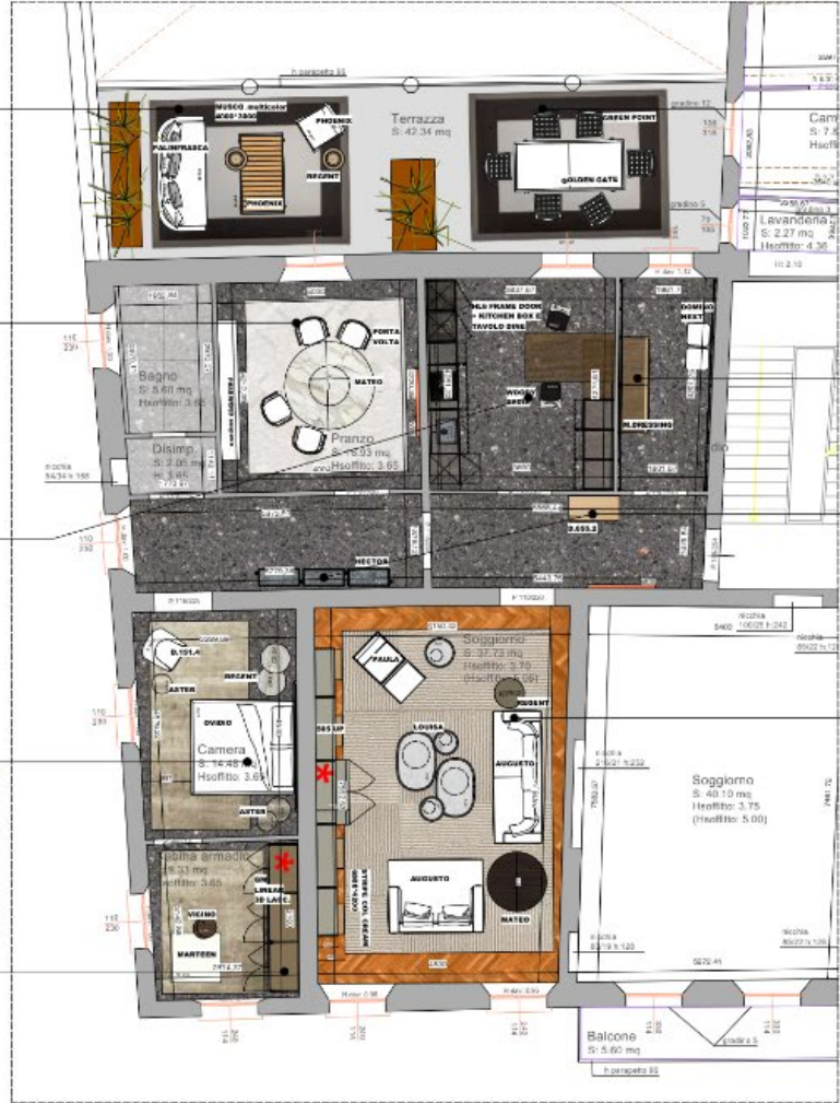
pianta 1°PIANO_scala 1.50
